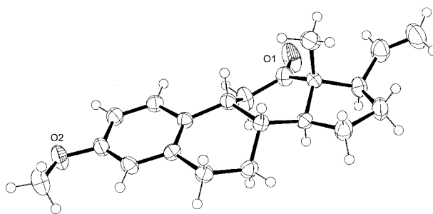
Figure 7. ORTEP diagram of steroid 9ad
